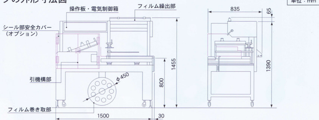
ASL250タイプの外形寸法図
